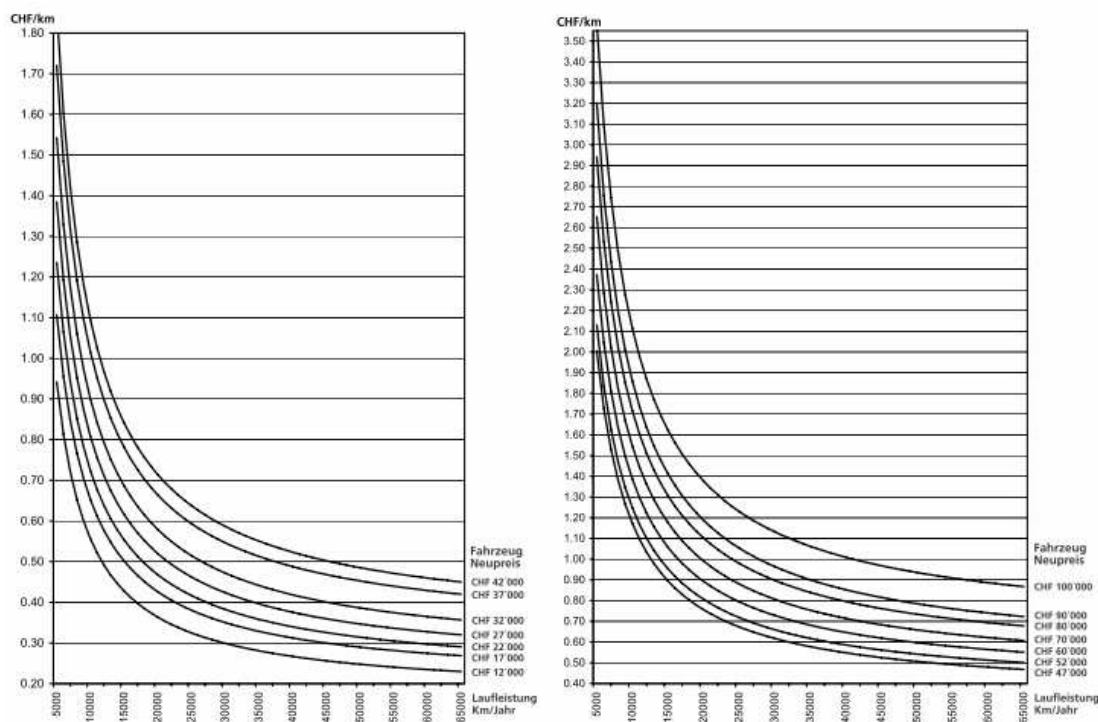
Illustration 3-1 : Coût du kilomètre dépendant du prix neuf de la voiture et du kilométrage annuel
